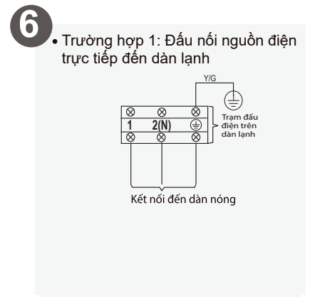
Đầu nối nguồn điện
