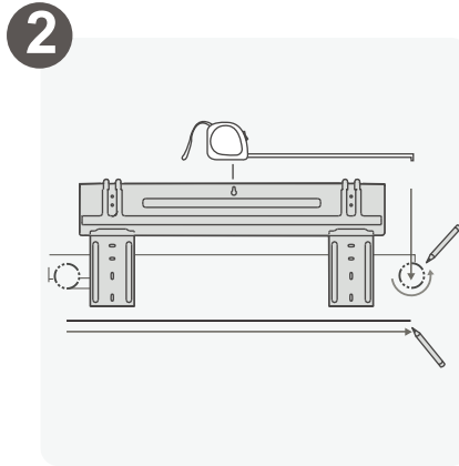
Xác định vị trí lỗ tường
