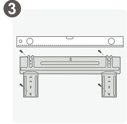
Lắp tấm treo tường
