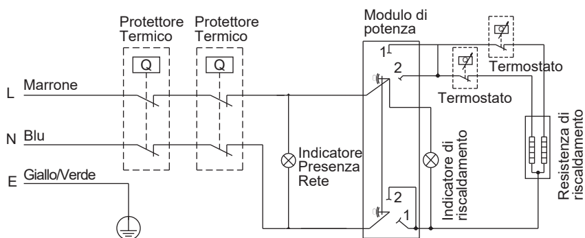
Schema elettrico
