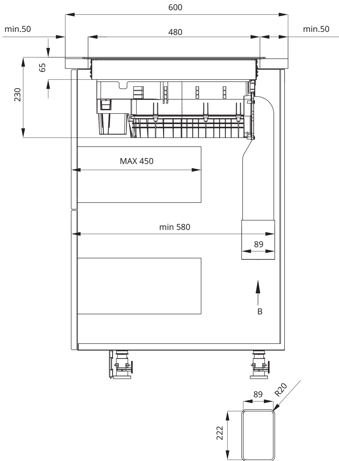
Ansicht: Adaptermaße
