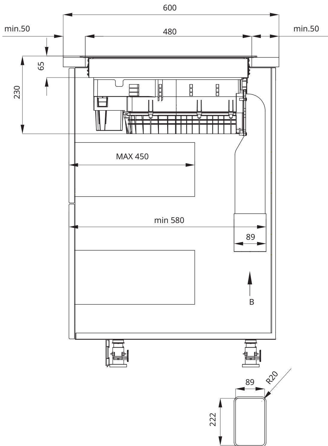
Vue : Dimension de l'adaptateur
