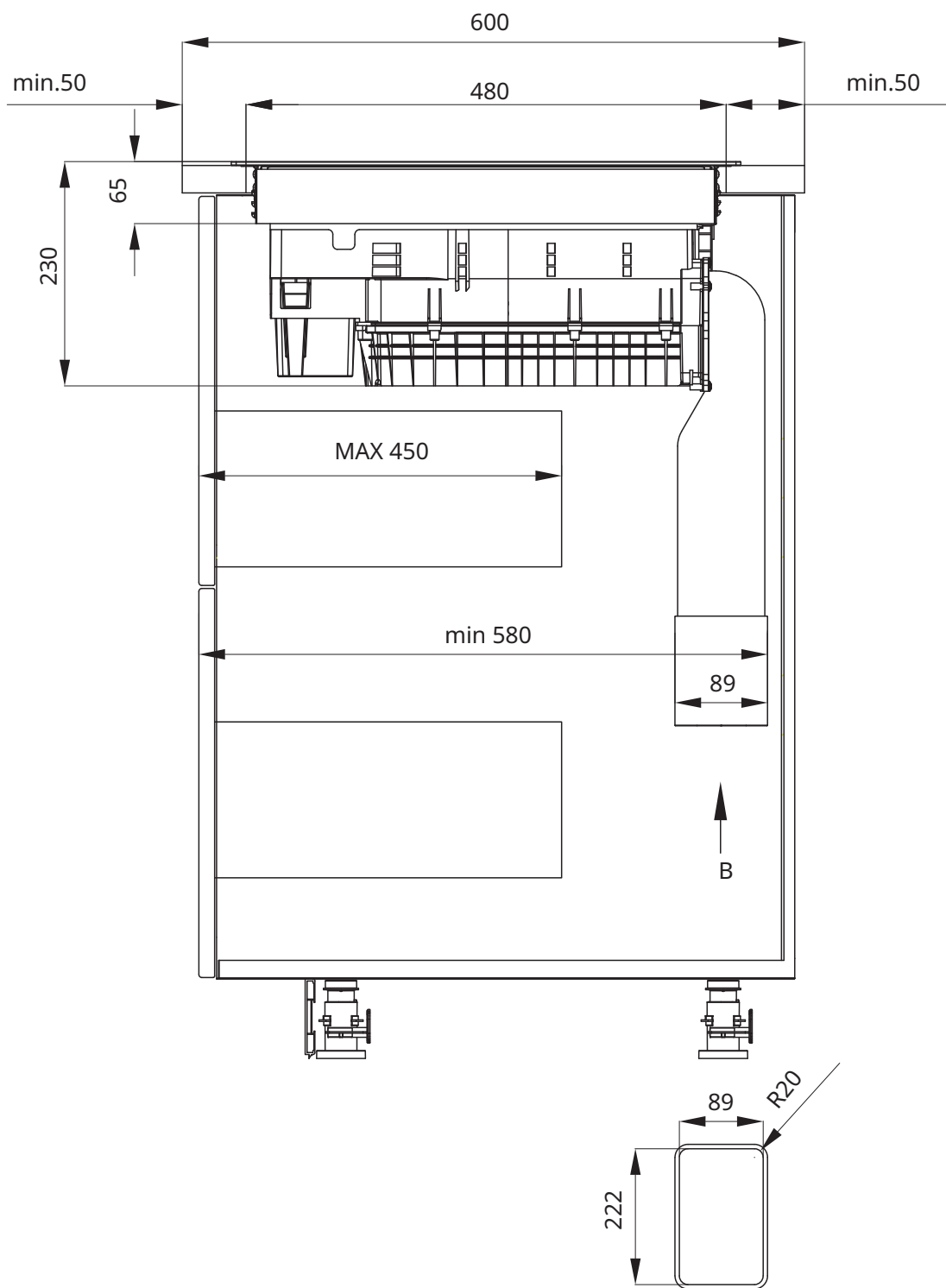
Vista: Dimensioni dell'adattatore
