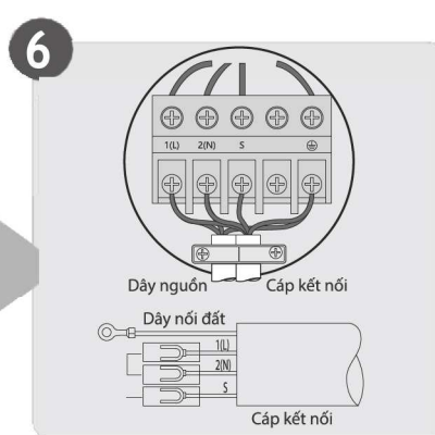
Kết nối dây điện
