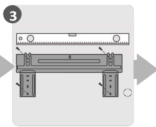
Gắn tấm kim loại
