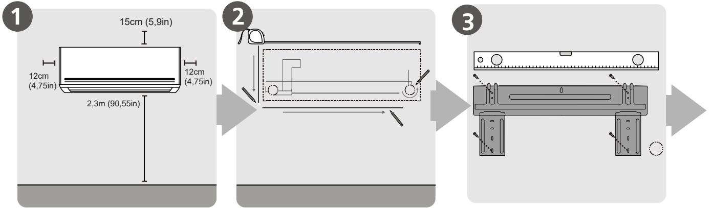
Lắp tấm treo tường
