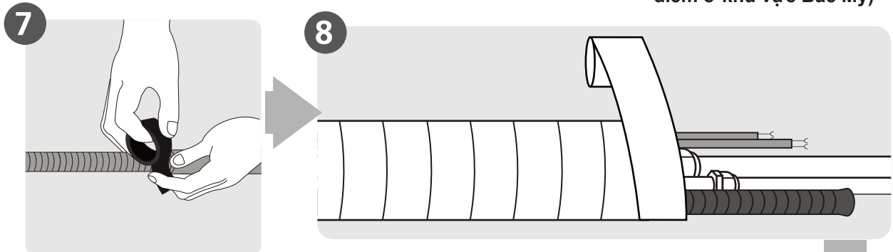
Bọc đường ống và cáp (không áp dụng cho một số địa điểm ở khu vực Bắc Mỹ)
